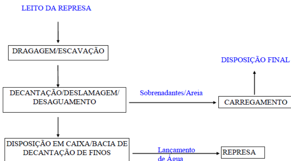
Figura 3. Fluxograma das operações no desassoreamento.
