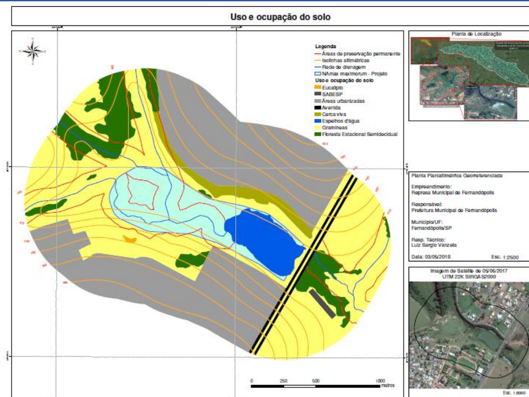
Figura 2. Detalhe da planta planialtimétrica do projeto de desassoreamento.
